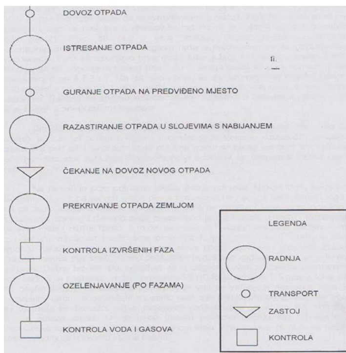
Slika 27. Tehnološka šema odlaganja otpada na RDM
