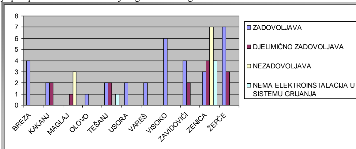
Grafikon 3.8. Stanje elektroinstalacija u sistemu grijanja srednjih škol (prikaz po općinama)
